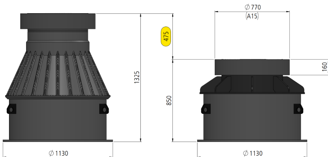
Höhenvergleich Typ M mit A15- Deckel: Standard zu COMPACT
