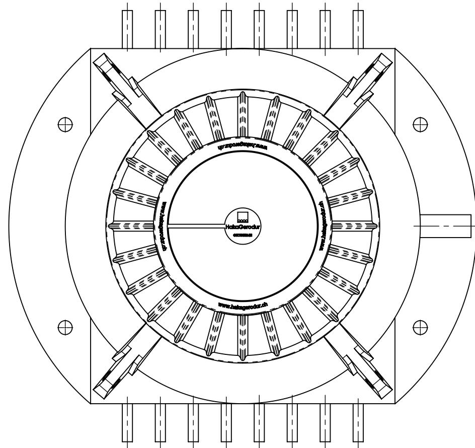
Kunststoffdeckel 200kg Couvercle en plastique 200kg Coperchio in plastica 200kg Plastic cover 200kg
