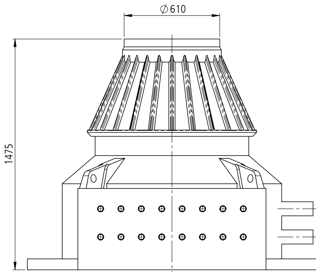
Ohne Abdeckung Sans Couvercle Sensa Copertura Without Cover
