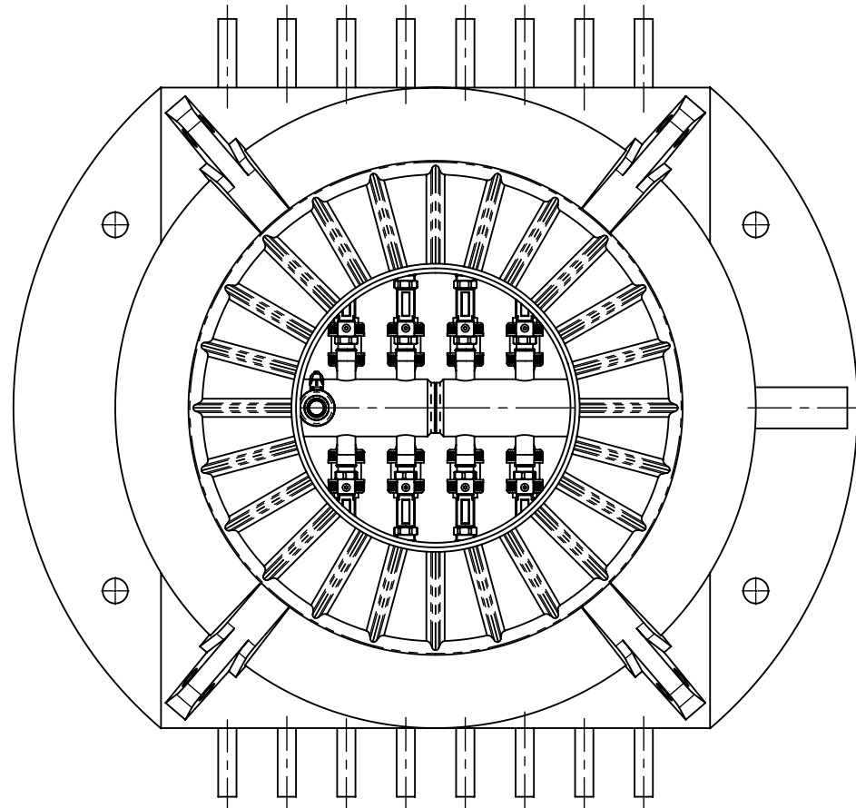
Ohne Abdeckung Sans Couvercle Sensa Copertura Without Cover
