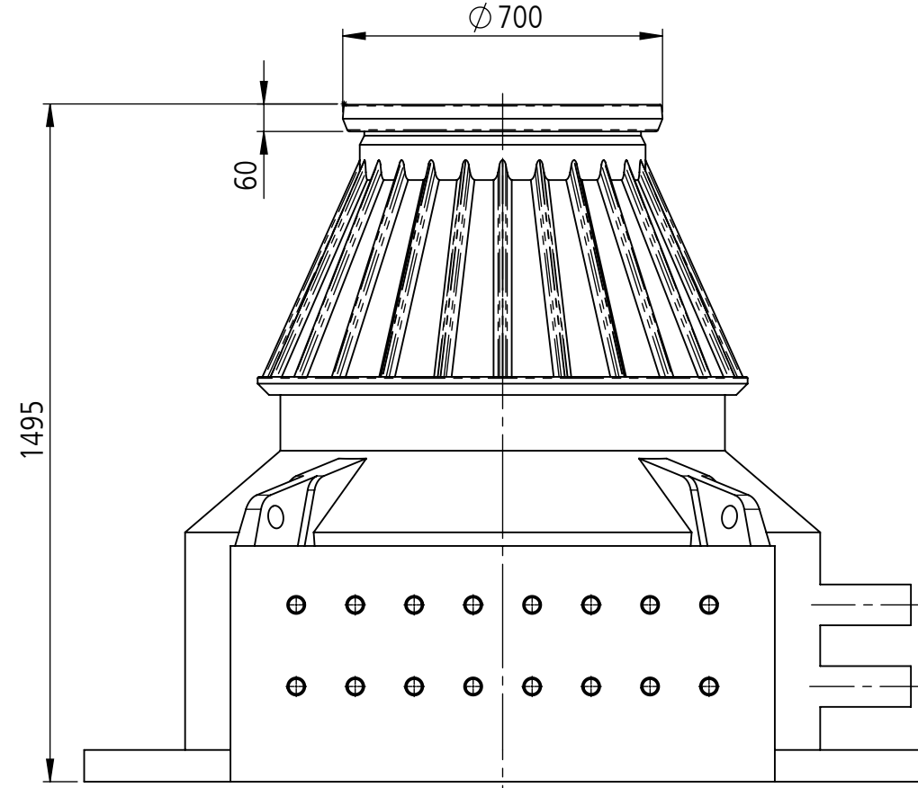
Kunststoffdeckel 200kg Couvercle en plastique 200kg Coperchio in plastica 200kg Plastic cover 200kg
