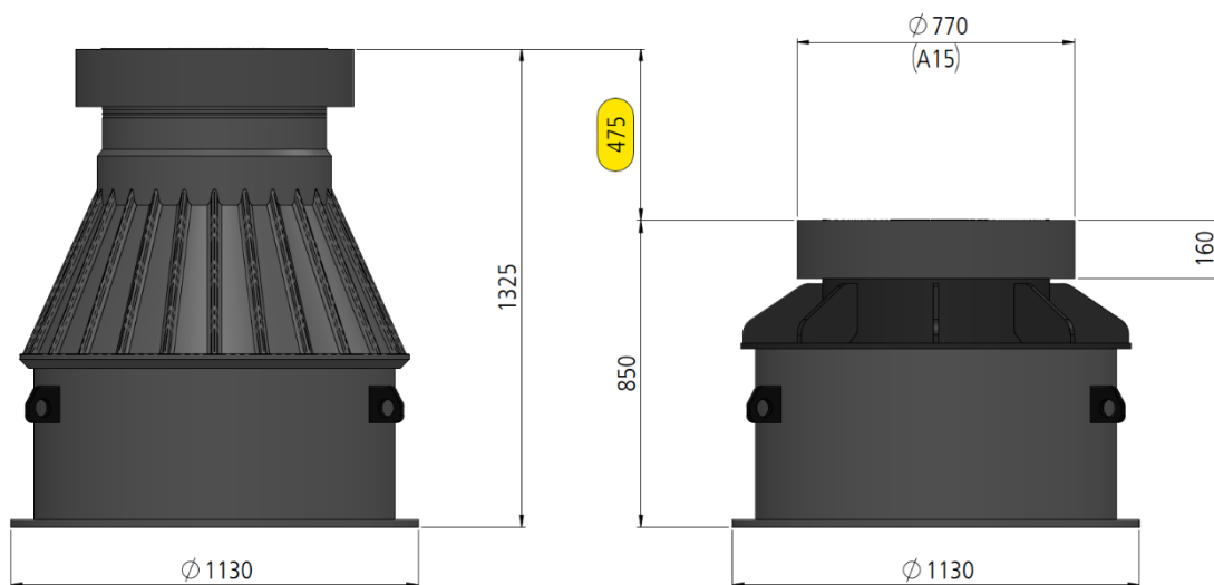
Comparaison des hauteurs, type M avec couvercle A15: standard et COMPACT
